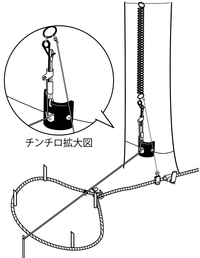
ワナの全体図
